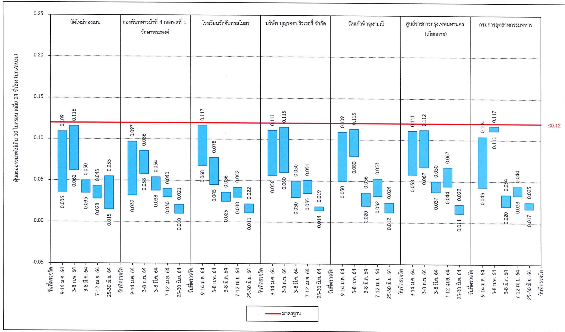
รูปที่ 3-8 ผลการติดตามตรวจสอบฝุ่นละอองขนาดไม่เกิน 10 ไมครอน เฉลี่ย 24 ชั่วโมง บริเวณสถานีติดตามตรวจสอบรอบโครงการ ระหว่างเดือนมกราคม-มิถุนายน พ.ศ. 2564
