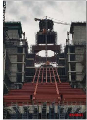
โครงสร้างเหล็ก Main Stair ฝั่งด้านหน้าอาคารหลัก
